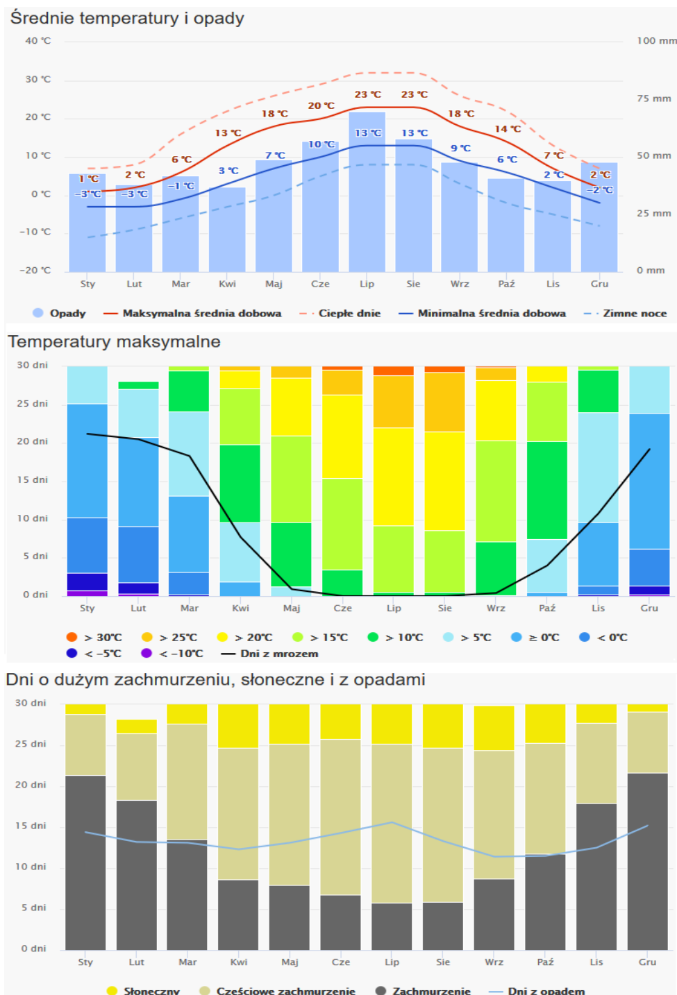
Rysunek nr 5. Warunki klimatyczne gminy Braniewo
