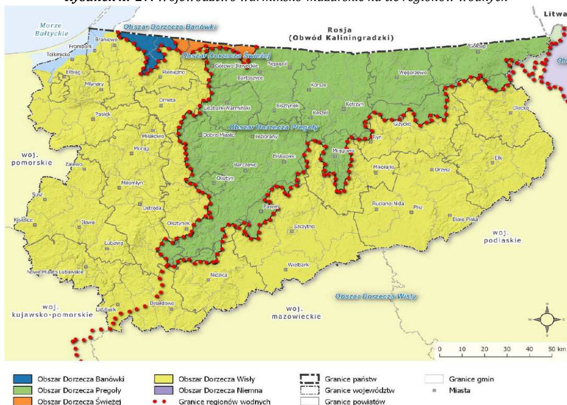
Rysunek nr 27. Województwo warmińsko-mazurskie na tle regionów wodnych
