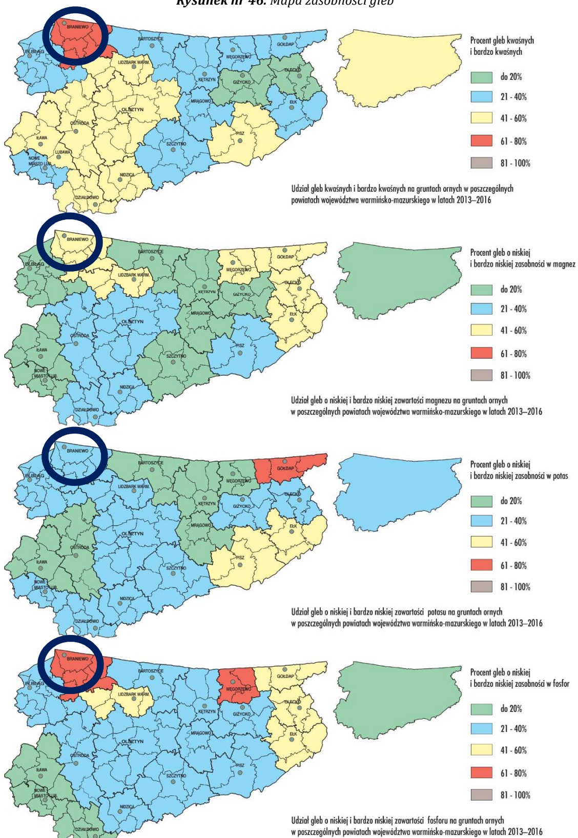
Rysunek nr 46. Mapa zasobności gleb
