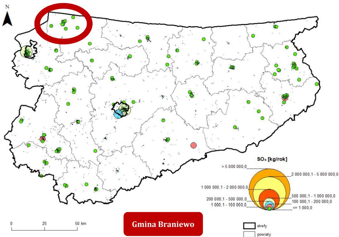
Rysunek nr 8. Lokalizacja punktowych źródeł emisji SO x na obszarze województwa warmińsko-mazurskiego
