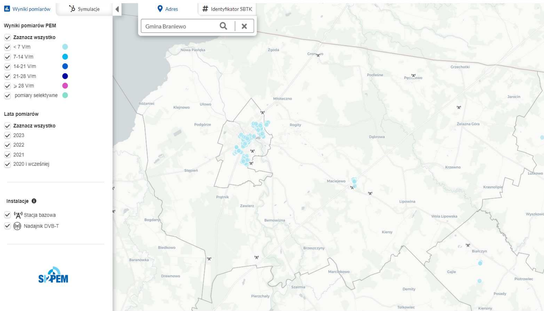
Rysunek nr 26. Lokalizacja gminy Braniewo względem stacji bazowych telefonii komórkowej i nadajników DVB-T oraz wyniki pomiarów PEM
