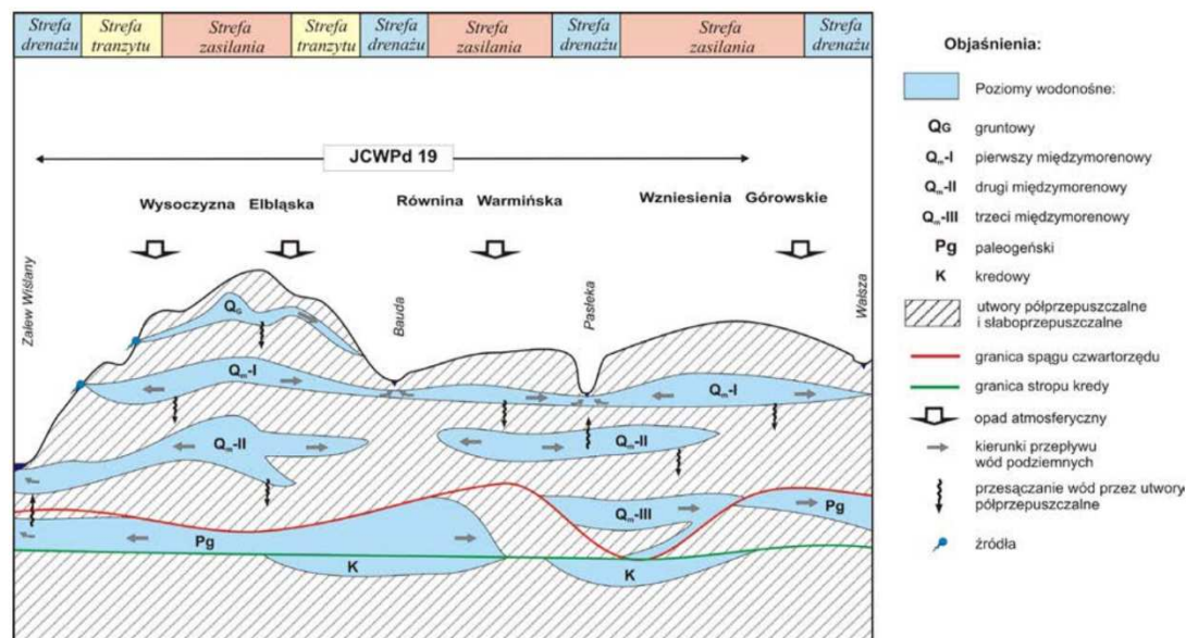
Rysunek nr 30. Charakterystyka JCWPd na terenie gminy Braniewo - JCWPd 19
