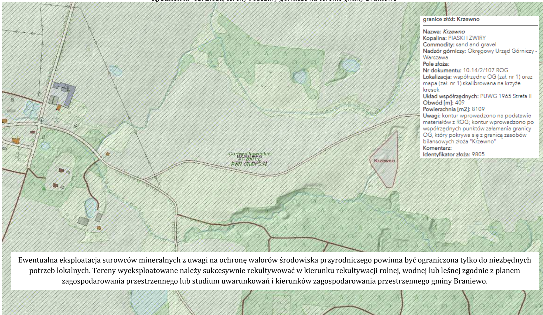
Rysunek nr 45. Złóża, tereny i obszary górnicze na terenie gminy Braniewo
