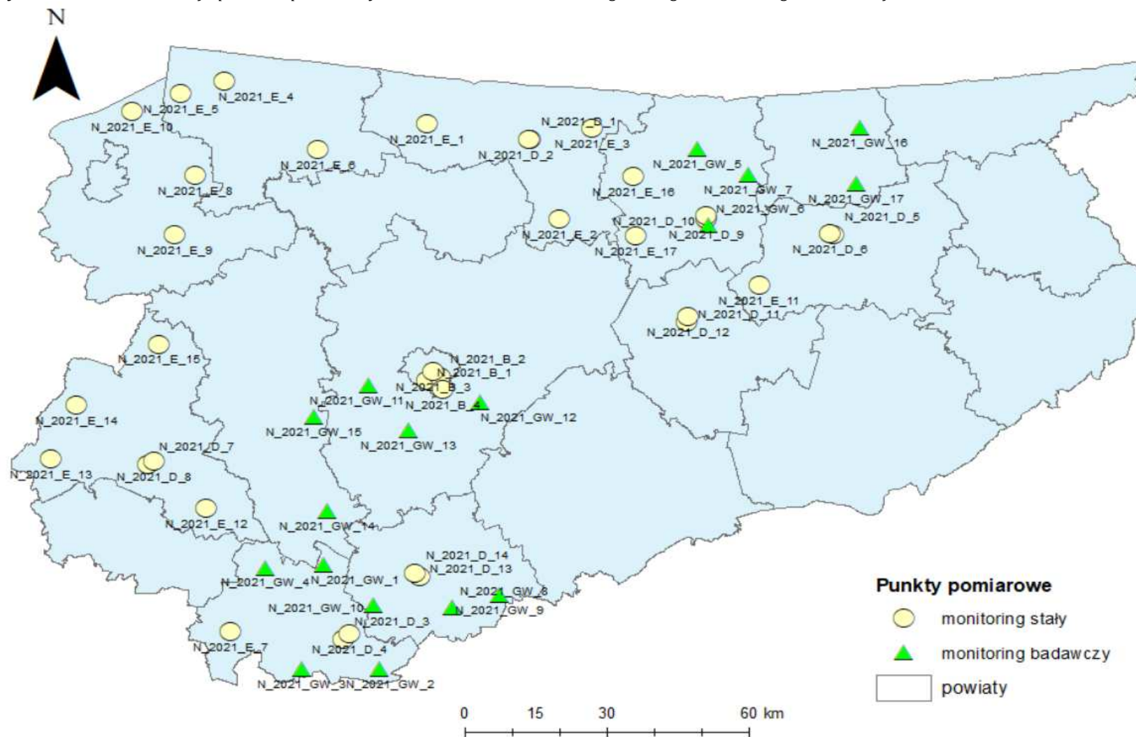
Rysunek nr 25. Lokalizacja punktów pomiarowych w 2021 roku dla monitoringu stałego i badawczego PEM w województwie warmińsko - mazurskim
