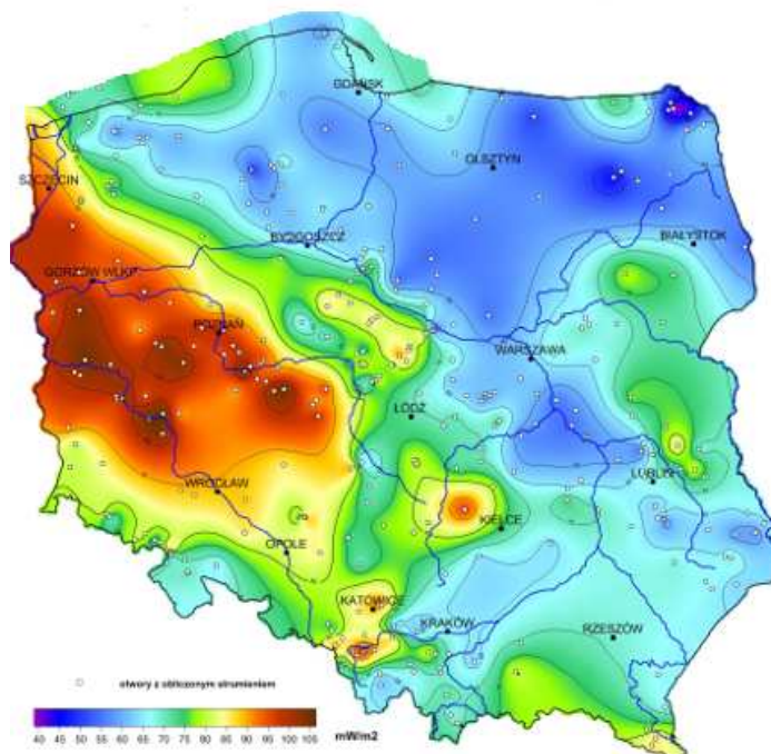
Rysunek nr 59. Mapa gęstości ziemskiego strumienia ciepłego dla obszaru Polski
