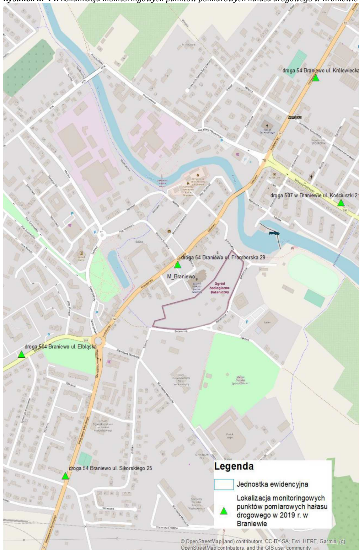
Rysunek nr 14. Lokalizacja monitoringowych punktów pomiarowych hałasu drogowego w Braniewie
