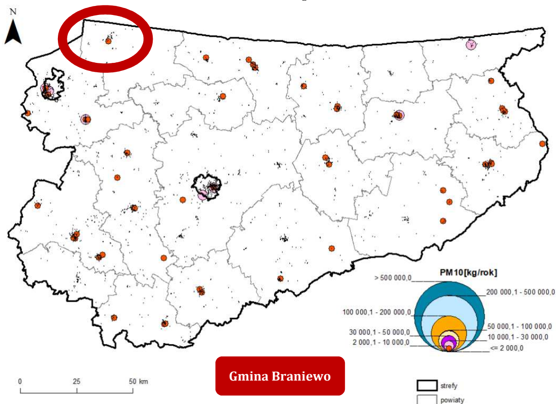
Rysunek nr 10. Lokalizacja punktowych źródeł emisji PM 10 na obszarze województwa warmińsko - mazurskiego
