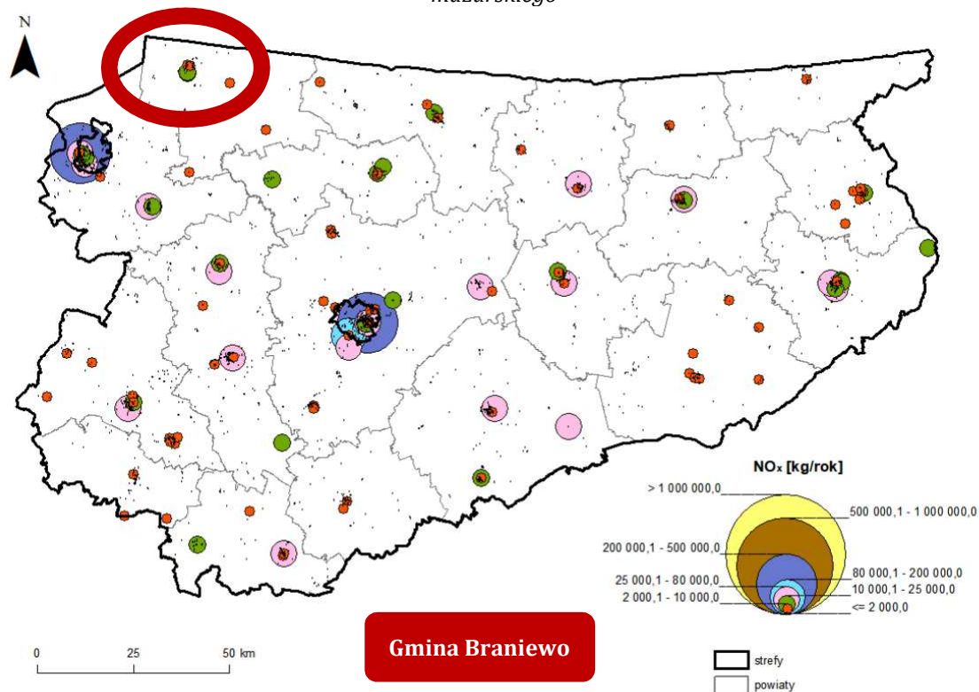
Rysunek nr 9. Lokalizacja punktowych źródeł emisji NO x na obszarze województwa warmińsko-mazurskiego
