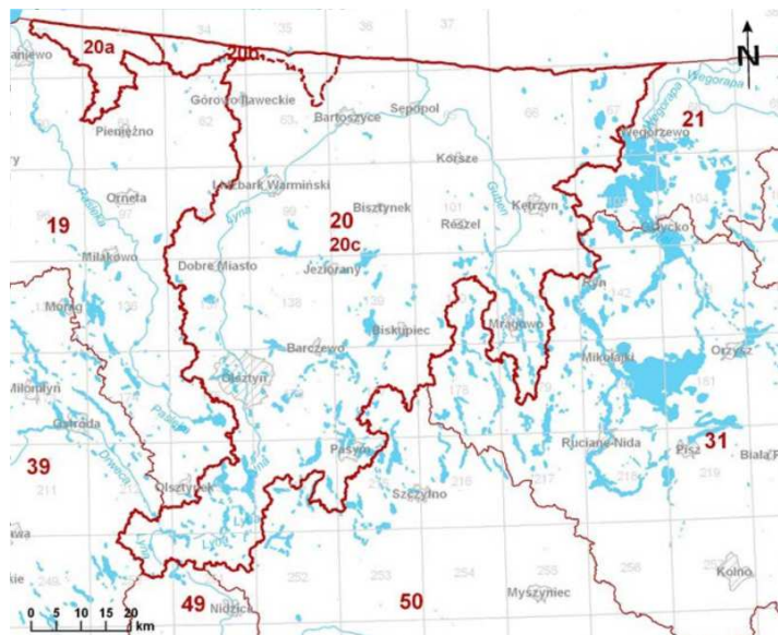
Rysunek nr 31. Charakterystyka JCWPd na terenie gminy Braniewo - JCWPd 20
