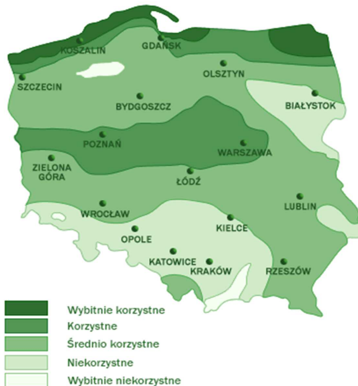
Rysunek nr 58. Mapa zasobów wietrznych IMIGW
