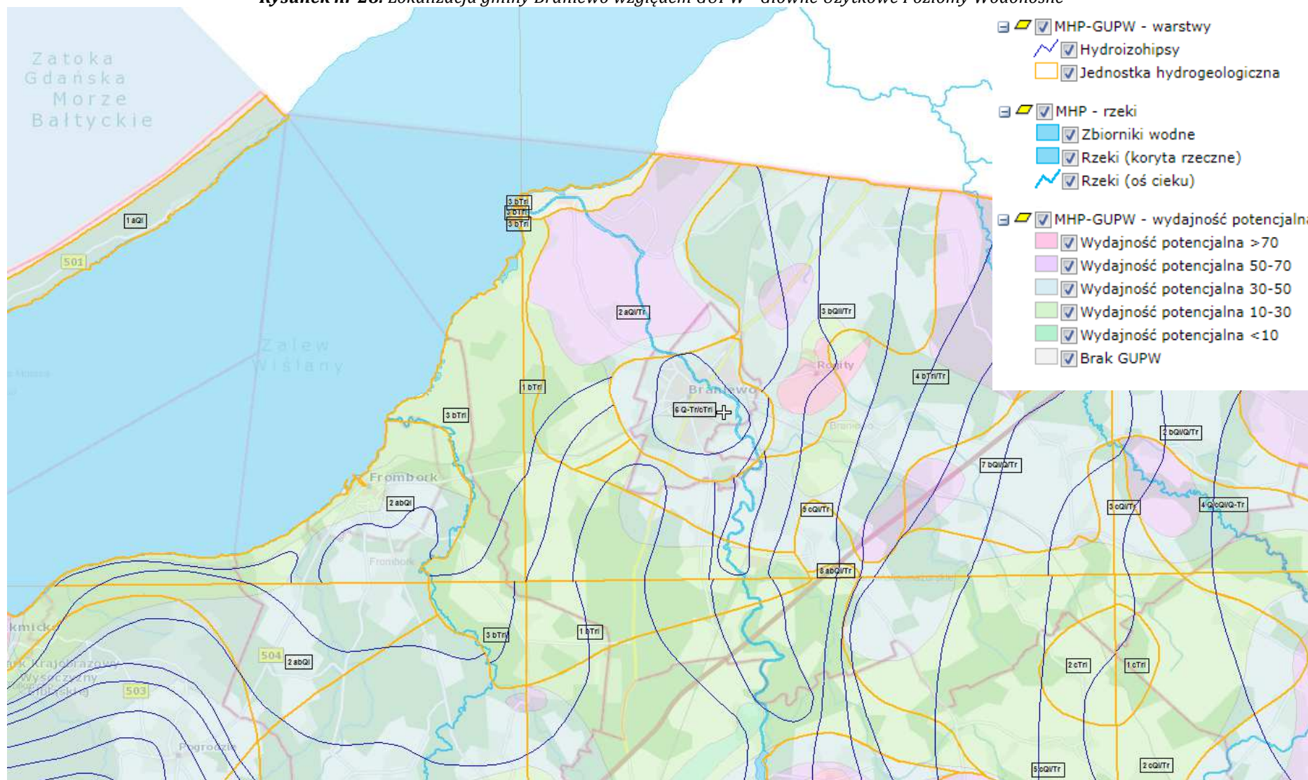
Rysunek nr 28. Lokalizacja gminy Braniewo względem GUPW - Główne Użytkowe Poziomy Wodonośne
