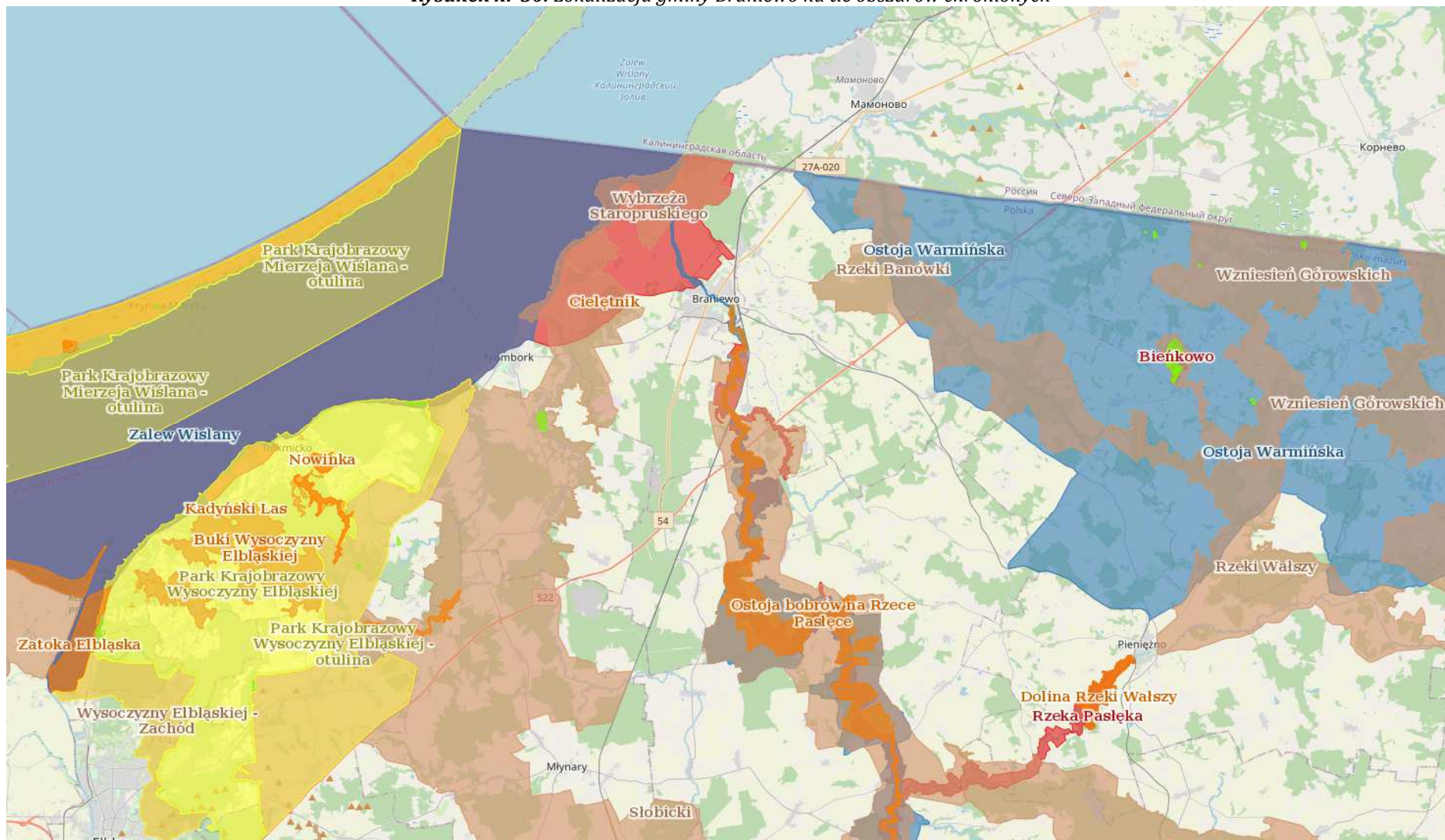
Rysunek nr 50. Lokalizacja gminy Braniewo na tle obszarów chronionych
